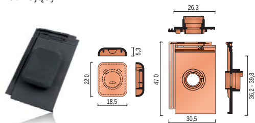
kominek odpowietrzający
