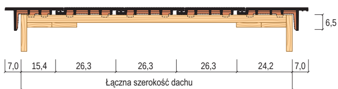
Detal krawędzi dachu z dachówkami szczytowymi
