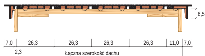
Detal krawędzi dachu z dachówkami szczytowymi połówkowymi.
