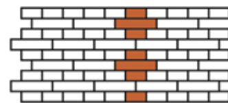
Крестовая кладка
