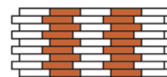
Ложковая кладка
