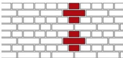
Крестовая. Тип I
