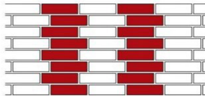
Ложковая в четверть кирпича
