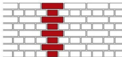
Крестовая. Тип II
