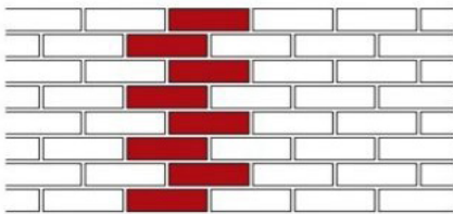
Ложковая в полкирпича
