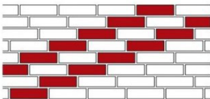
Ложковая диагональная со сдвигом в четверть кирпича
