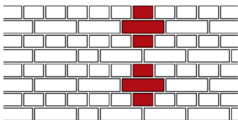
Крестовая. Тип I
