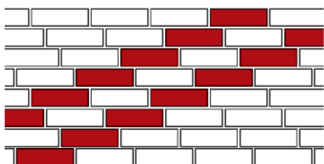
Ложковая диагональная со сдвигом в четверть кирпича
