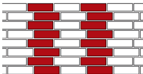
Ложковая в четверть кирпича
